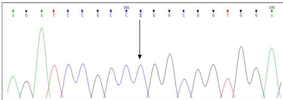
شکل (۲): نتیجه تعیین توالی ژن mexZ پیکان سیاه‌رنگ تغییر باز G در موقعیت ۴۲۸ به C را نشان می‌دهد که باعث تبدیل آمینواسید آرژنین به پرولین در کدون CGG(Arg) > CCG(Pro) در کدون ۱۴۳ این ژن (R143P) شد.
