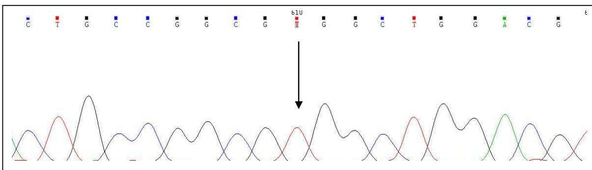
شکل (۴): نتیجه تعیین توالی ژن mexZ پیکان سیاه‌رنگ، تغییر باز C در موقعیت ۴۵۷ به T را نشان می‌دهد که باعث تبدیل آمینواسید آرژنین به تریپتوفان در کدون CGG(Arg) > TGG(Trp) در کدون ۱۵۳ این ژن (R153W) شده است.
