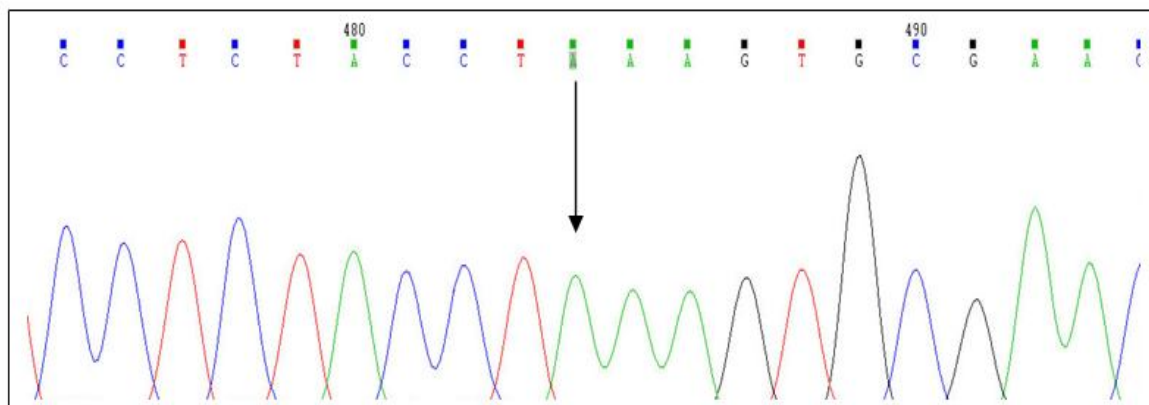
شکل (۳): نتیجه تعیین توالی ژن mexZ پیکان سیاه‌رنگ تغییر باز C در موقعیت ۳۳۳ به A را نشان می‌دهد که باعث تبدیل آمینواسید لوسین به گلوتامیک اسید در کدون CTC(Leu) > CTA(Glu) در کدون ۱۱۱ این ژن (L111E) شده است.
