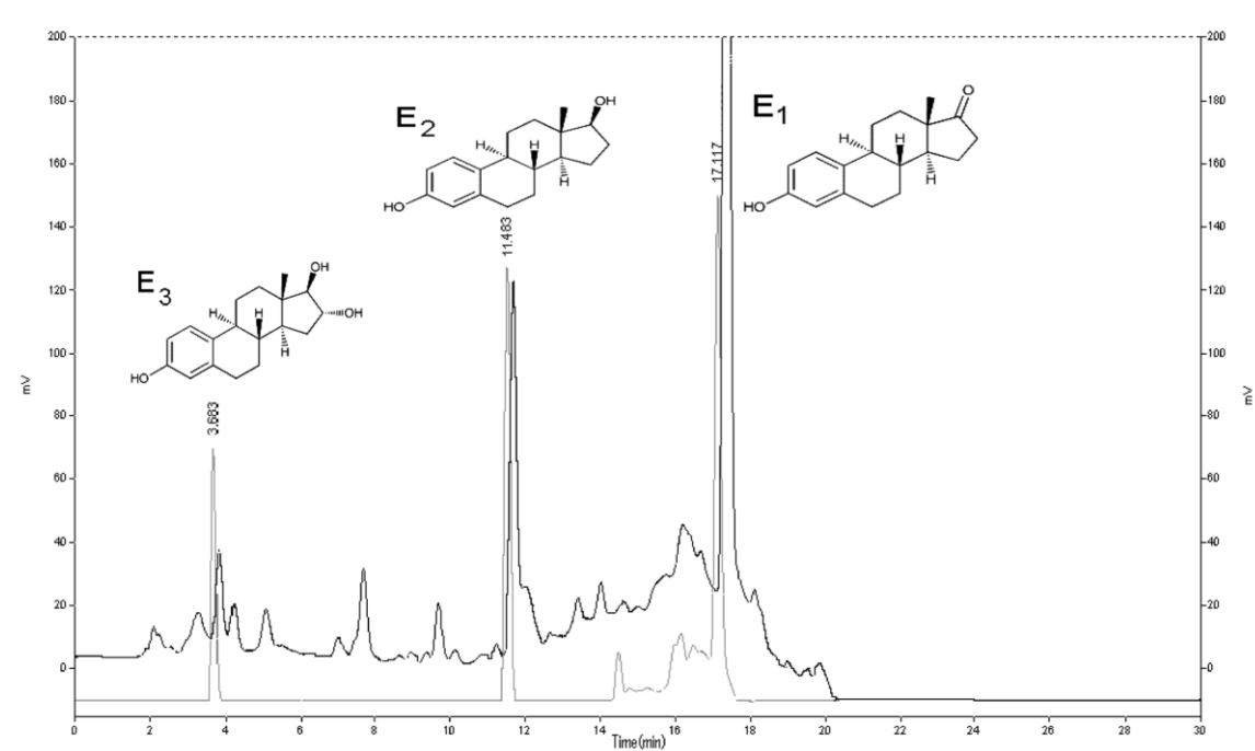
کروماتوگرام شماره (9): کروماتوگرام HPLC مربوط به E1، E2 و E3: کروماتوگرام تیره استروژن‌ها را در شیر و کروماتوگرام روشن استروژن‌ها را در محلول استاندارد نشان می‌دهد. E1: استرون، E2 17β به تا-استرادیول و E3: استریول
